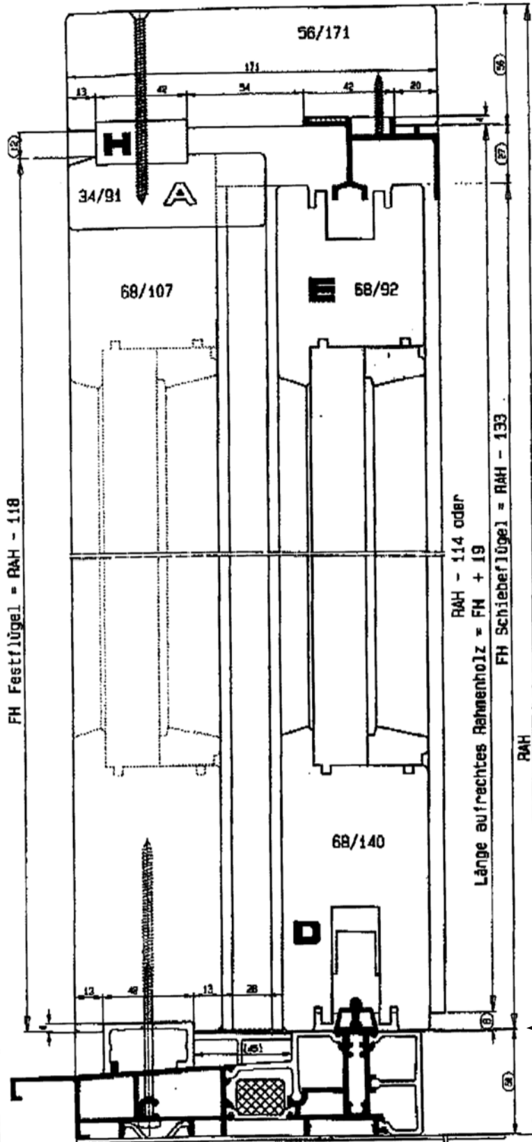
Vertikalschnitt Schema A, C, G und K 20 mm Flügelabstand
