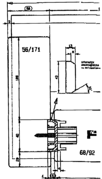
Horizontalschnitt Schema A 20 mm Flügelabstand
